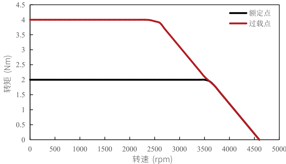
T-N曲线
